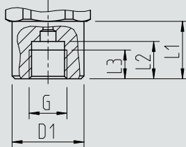
EN 837, rosca fêmea
